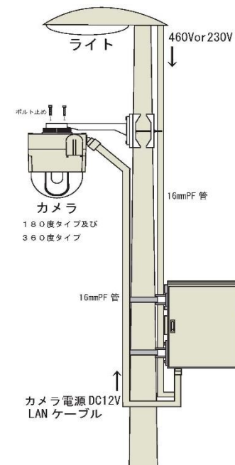
道路監視カメラ・レコーダー・取付概念図
