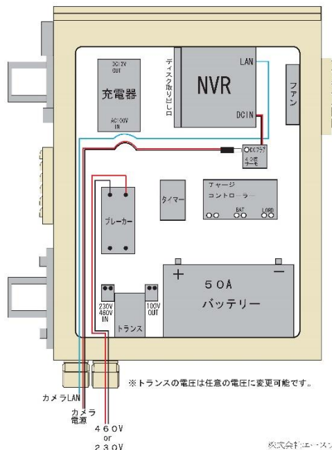
道路監視用レコーダー BOX 配線概念図
